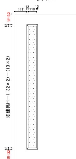
採光A
