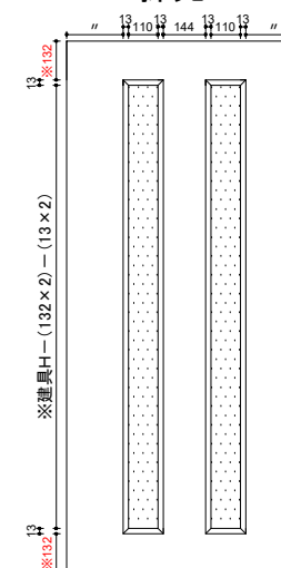
採光H
