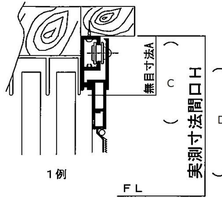
(ランマなし縦断面図)
