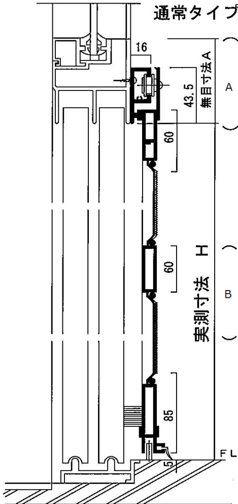
(ランマ付縦断面図)
